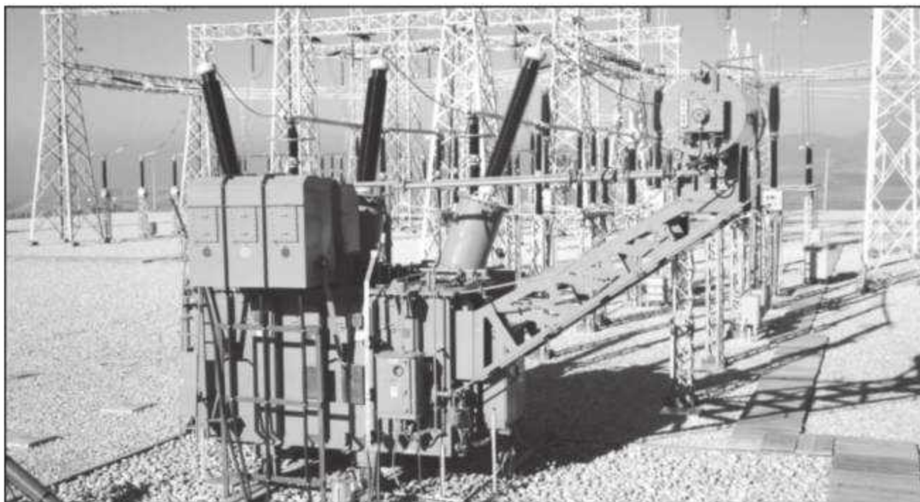
अयबक सब स्टेशन, अफगानिस्तान में 16 एम वी ए पावर ट्रांसफोर्मर
